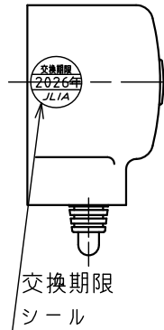
A矢視図
